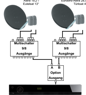
Beispiel 3: 4 Satelliten (Quattro-LNBs) Astra 19,2°/ Eutelsat 13° Eurobird-Astra 28,5°/ Türksat 42°
